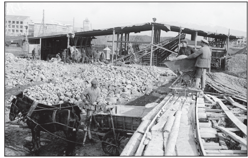
Երևանի բետոնի գործարանի շինարարությունը, 1935 թ.
